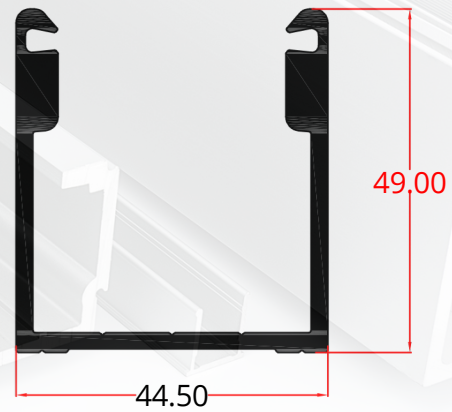
TGN 1001
