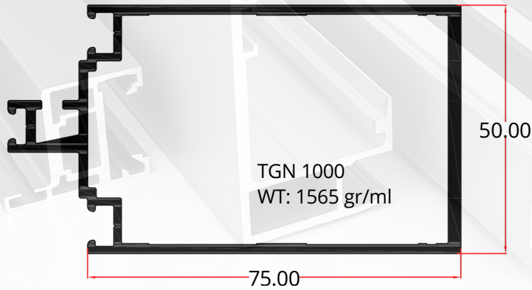
TGN 1000
